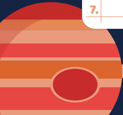
Jupiter
