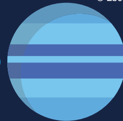
Neptun
