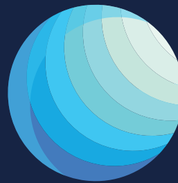
Uran
