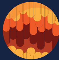
Venera
